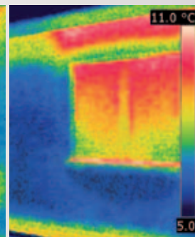
Beispiel: Heizkörpernische NACH der Dämmung
