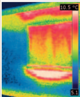
Beispiel: Heizkörpernische VOR der Dämmung
